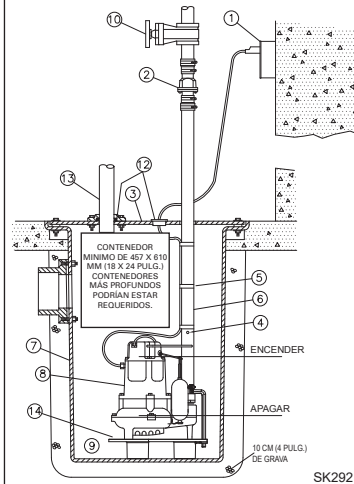
INSTALACIÓN TÍPICA PARA ACHIQUE
