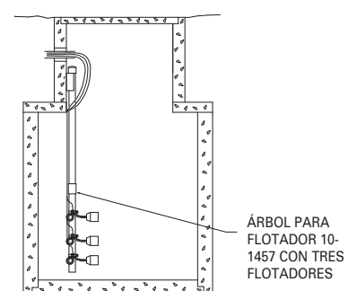
SOPORE COLGANTE PARA FLOTADOR TÍPICO EN FOSOS DE CONCRETO O TUBOS VERTICALES PARA TANQUES SÉPTICOS
