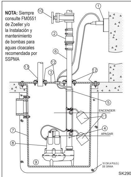
INSTALACIÓN TÍPICA PARA AGUAS NEGRAS
