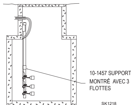
SUPPORT DE FLOTTES TYPIQUE POUR PUISARD EN BÉTON OU POUR PUITS D'ACCÈS DE FOSSE SEPTIQUE
