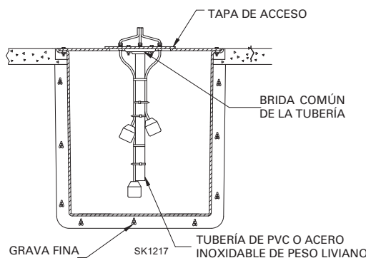
SOPORE COLGANTE PARA FLOTADOR TÍPICO EN FOSOS CON TAPA DE ACERO
