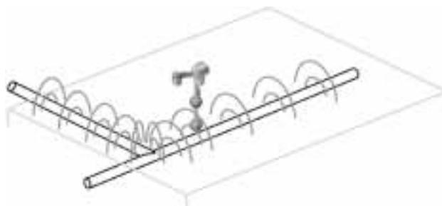
Figure 2 – Champ composite au droit d'une connexion de ligne.
